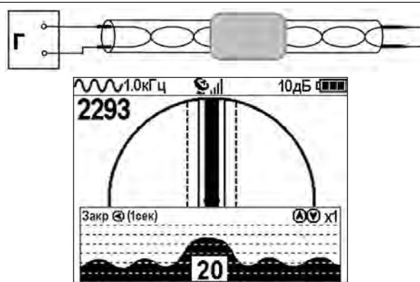
Рис.А.2 Муфта
